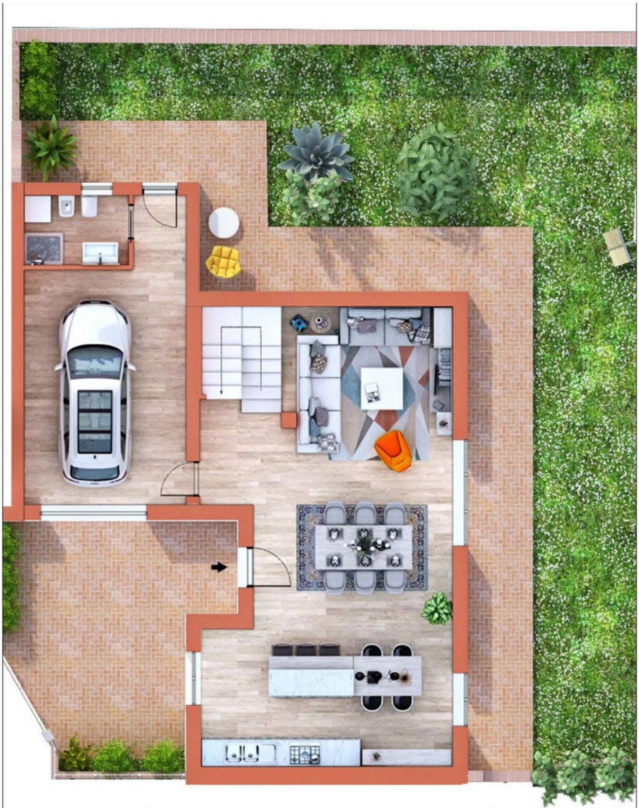
UNITA' ABITATIVA n° 2 PIANTA PIANO TERRA (QUOTA +0,00) SCALA 1:50
