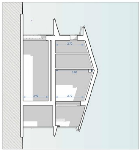
Sezione E-E
