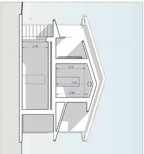
Sezione D-D
