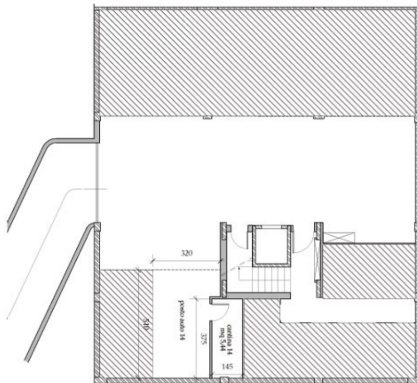
PIANTA PIANO SEMINTERATO - SCALA 1:100
